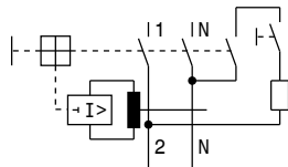
Fehlerstromschutzschalter
