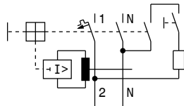
Fehlerstrom- Leitungsschutzschalter kombiniert
